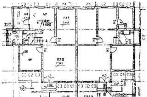
豪华别墅面积200—250M 2 （底层车库、室内装饰用户自订、前后庭院）
