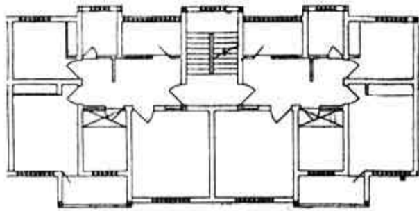
80型住宅（南客北餐）
